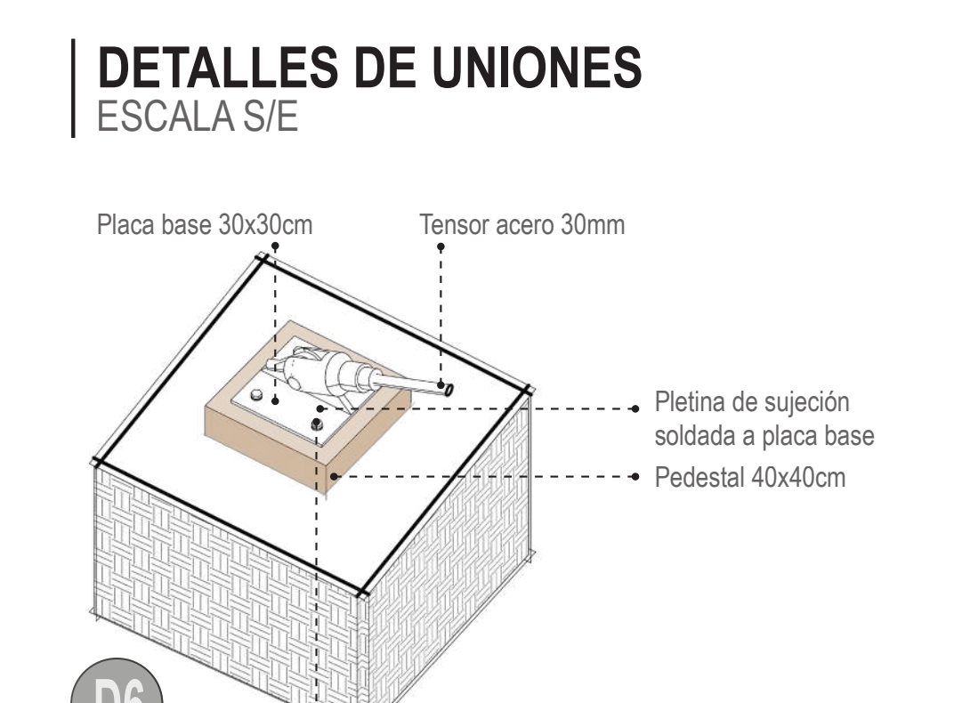
D5 DETALLE ESTRUCTURA CONTRAPUESTA ESCALA S/E
