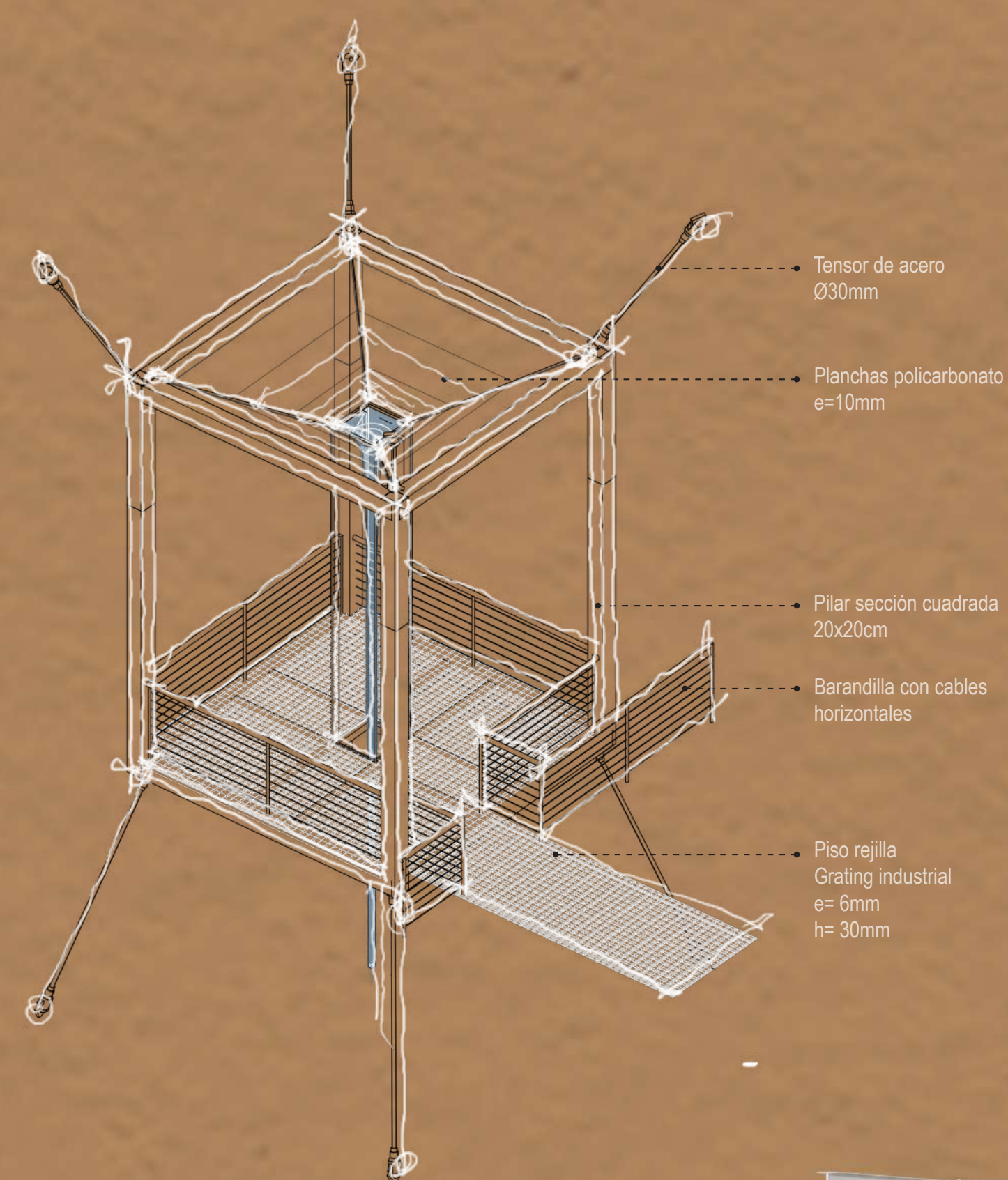
DETALLE MIRADOR ESCALA S/E
