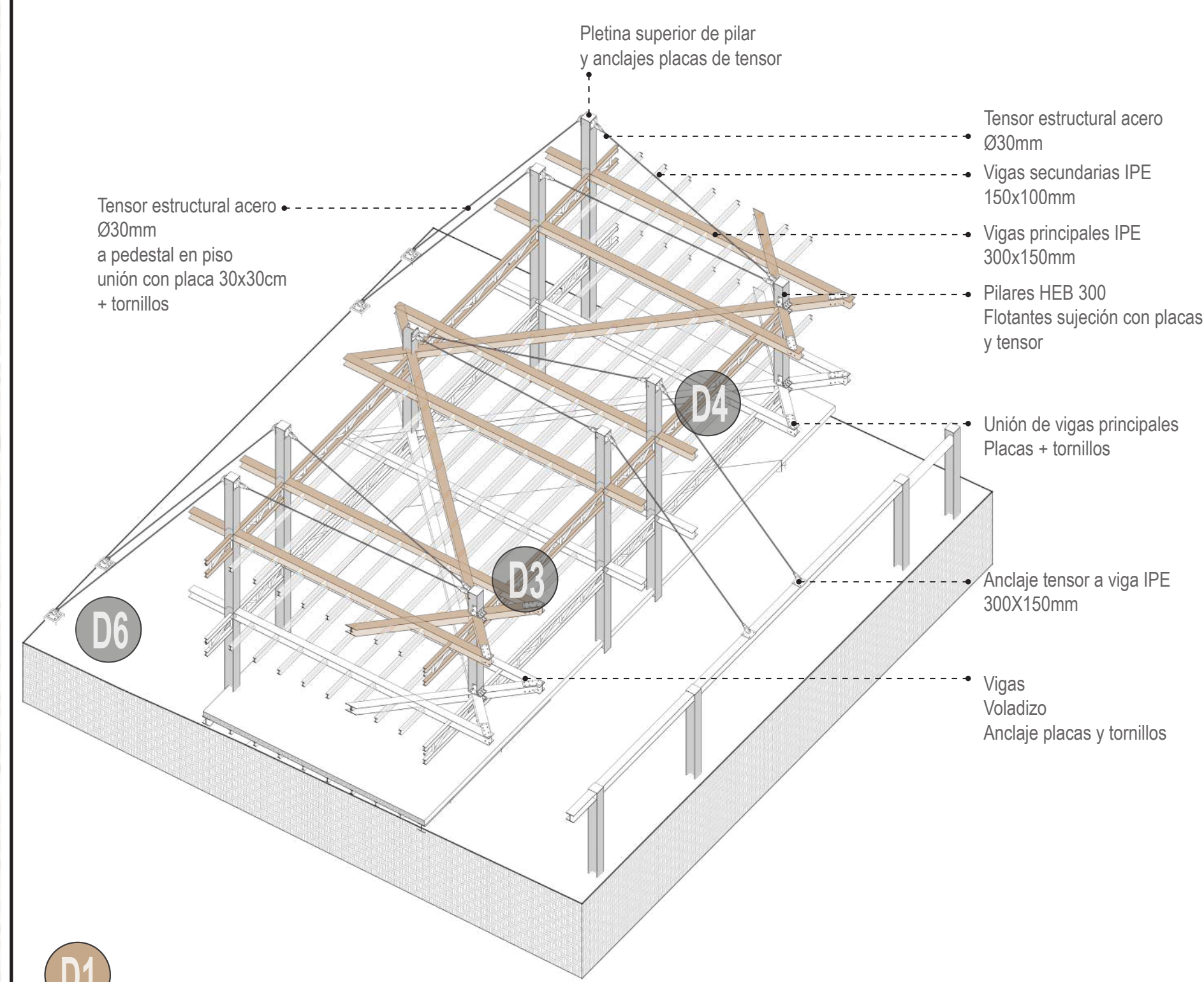
D1 DETALLE ESTRUCTURA CONTRAPUESTA ESCALA S/E
