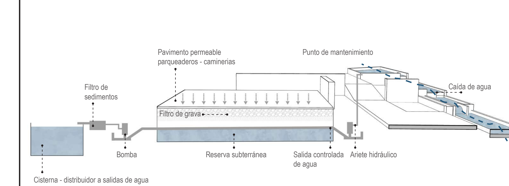
ESQUEMA TRATAMIENTO DE AGUA LLUVIA ESCALA S/E
